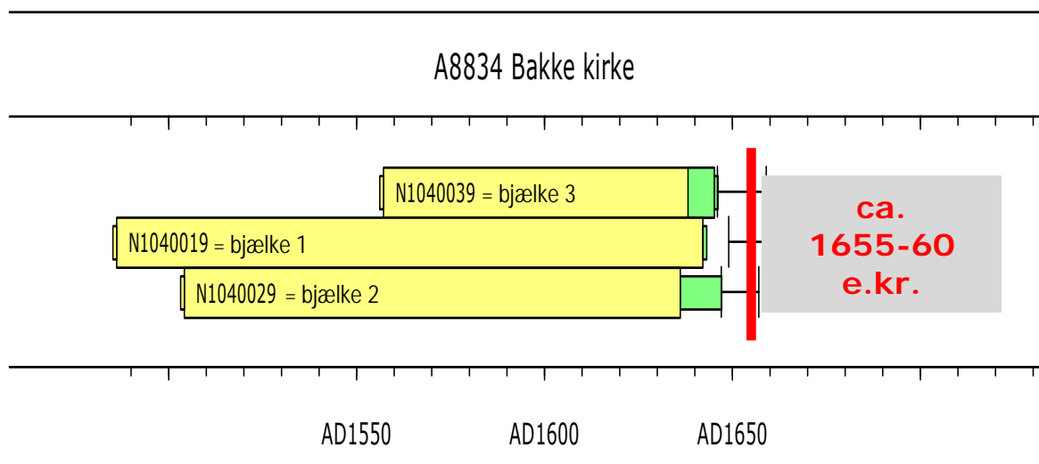
Figur 1: Dateringsdiagram. Tømmer fra Bakke kirke, Flekkefjord kommune. Indplacering af de daterede prøver på en tidsskala. (Den grønne signatur angiver bevaret splintved.)
