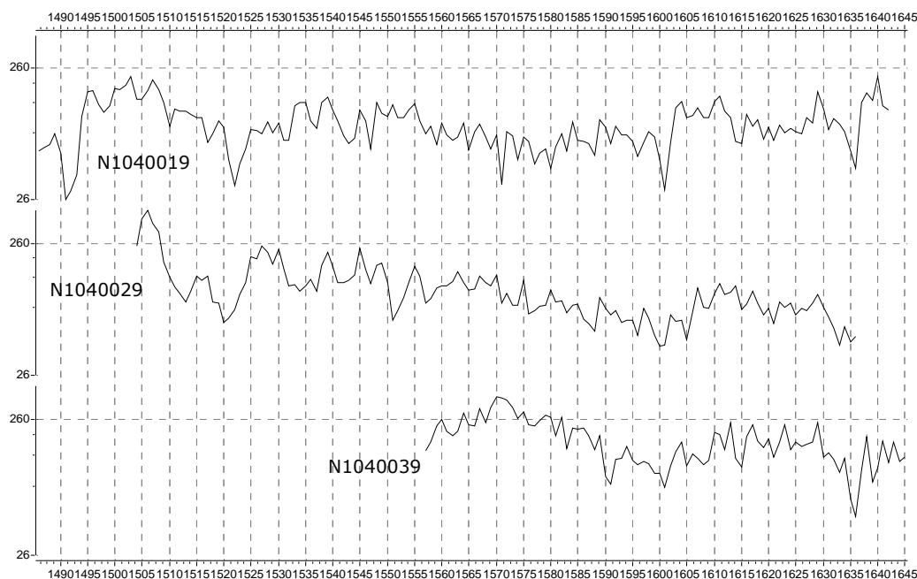
Figur 2: Dateringsdiagram. Tømmer fra Bakke kirke, Flekkefjord kommune. Indplacering af de daterede årringskurver på en tidsskala.
